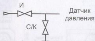
Рисунок А.2 – Клапанный блок БКН2
