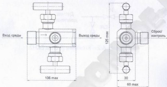
Рисунок Б.2 – Клапанный блок БКН2
