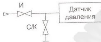
Рисунок А.2 – Клапанный блок БКН2
