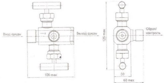
Рисунок Б.2 – Клапанный блок БКН2
